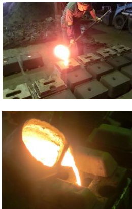
コシキと呼ばれる溶解炉で鉄を溶かす 鉄の溶解(1,400°C)
