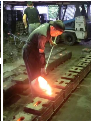
注湯(砂型に職人が一つ一つ溶解した鉄を流し込む) 鉄を途切れないよう温度が冷めないうちに注ぐ。
